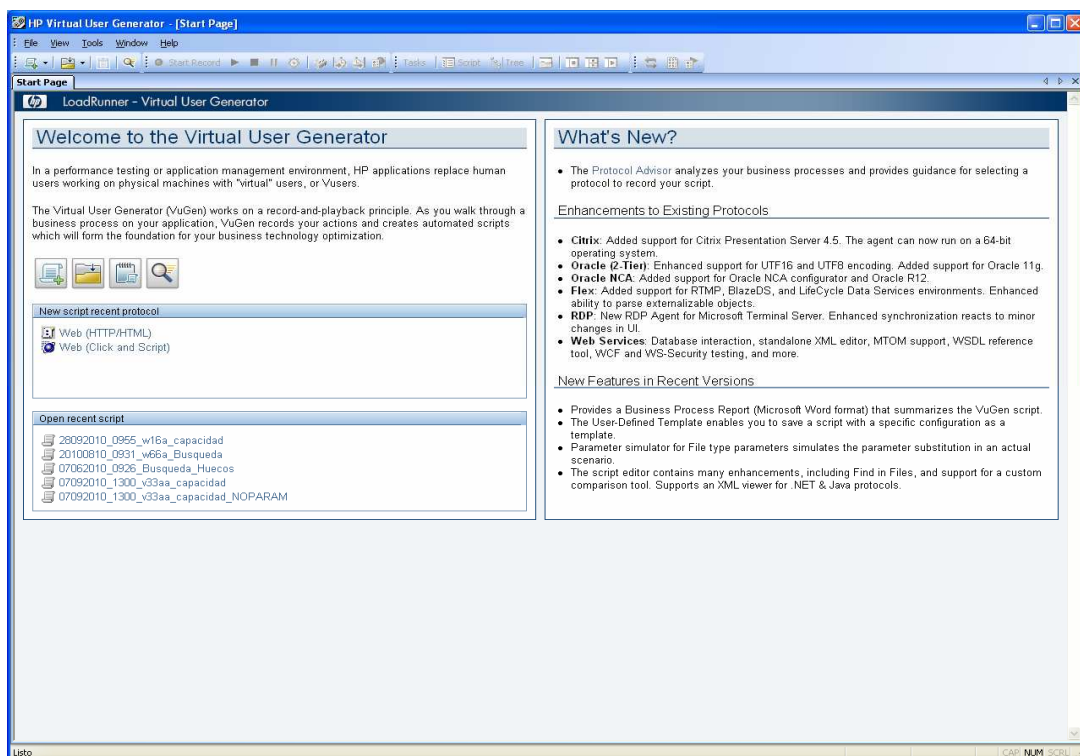
Figura 3: Inicio VuGen
