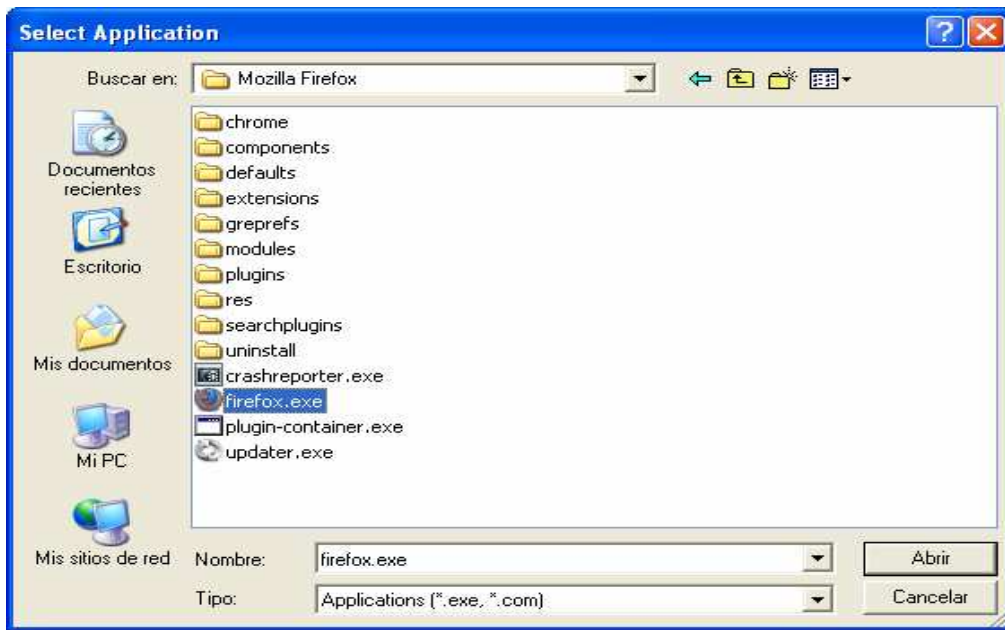
Figura 6: Selección carpeta
