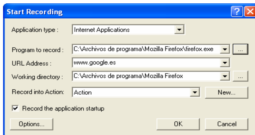
Figura 5: selección carpeta
